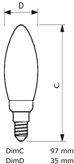
Abmessungsskizze
